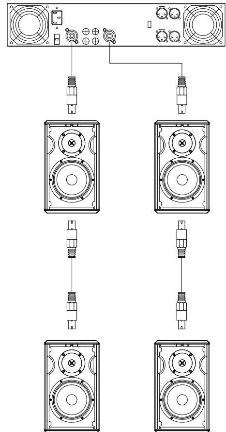
Fig. 3. Configuración Full-range estéreo en paralelo
