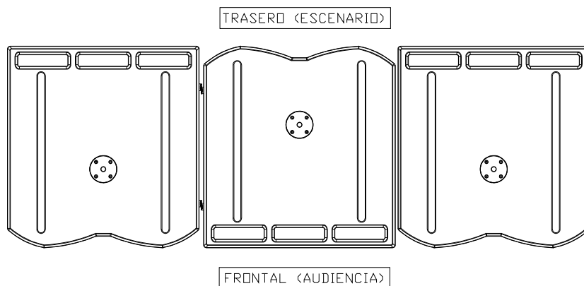
Fig. 3. Configuración cardiode básica para S218W
