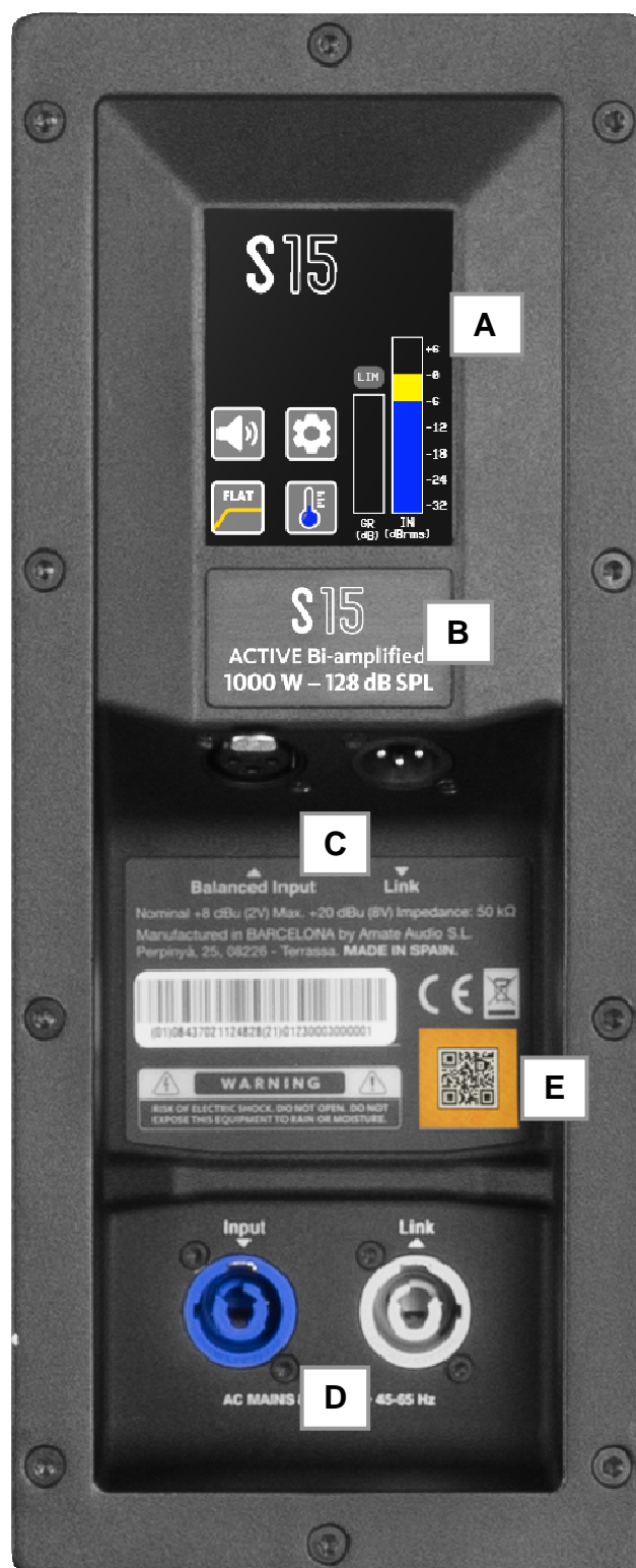
Fig. 2. Panel de control y conexiones de la S15
