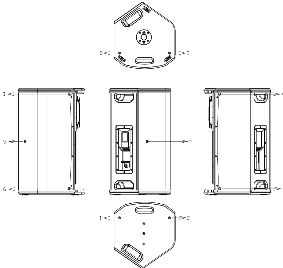
Fig. 15. Volado de una unidad S15 con ACR-M8
