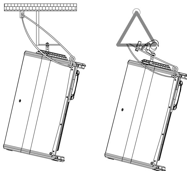
Fig. 13. Volado de una unidad S15 con HR-LU y HR-LU/GT
