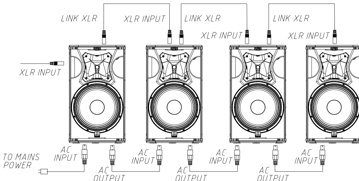
Fig. 3. Conexiones en paralelo para la S15
