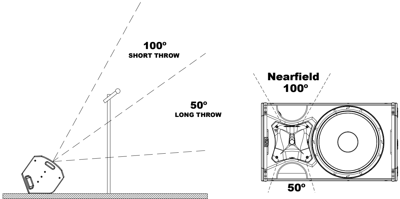
Fig. 10. Uso como monitor de escenario (caso 1)
