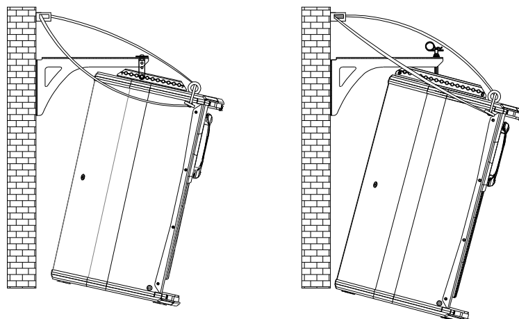
Fig. 14. Volado de una unidad S15 con SP-WHR
