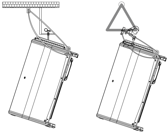
Fig. 17. Volado de una unidad S15 con RB-L y RB-L/GT
