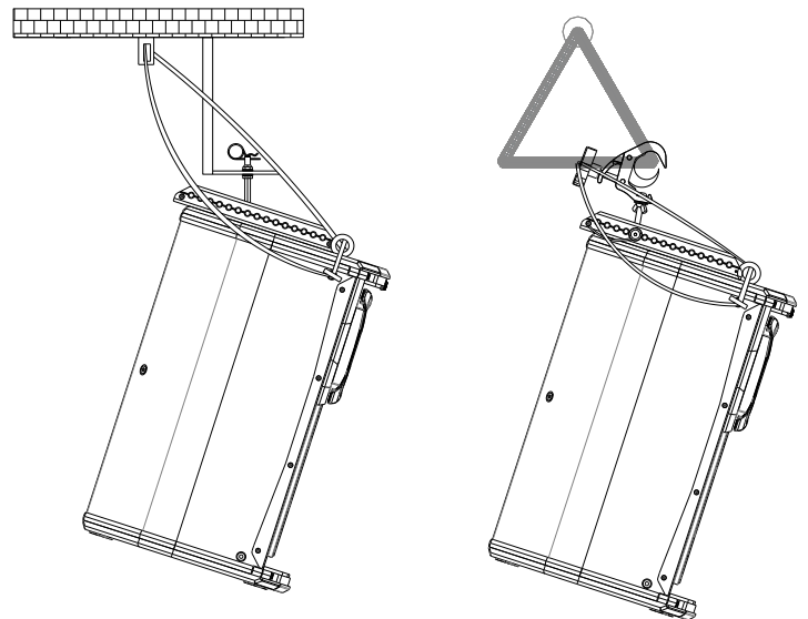
Fig. 14. Volado de una unidad S12A7 con RB-L y RB-L/GT
