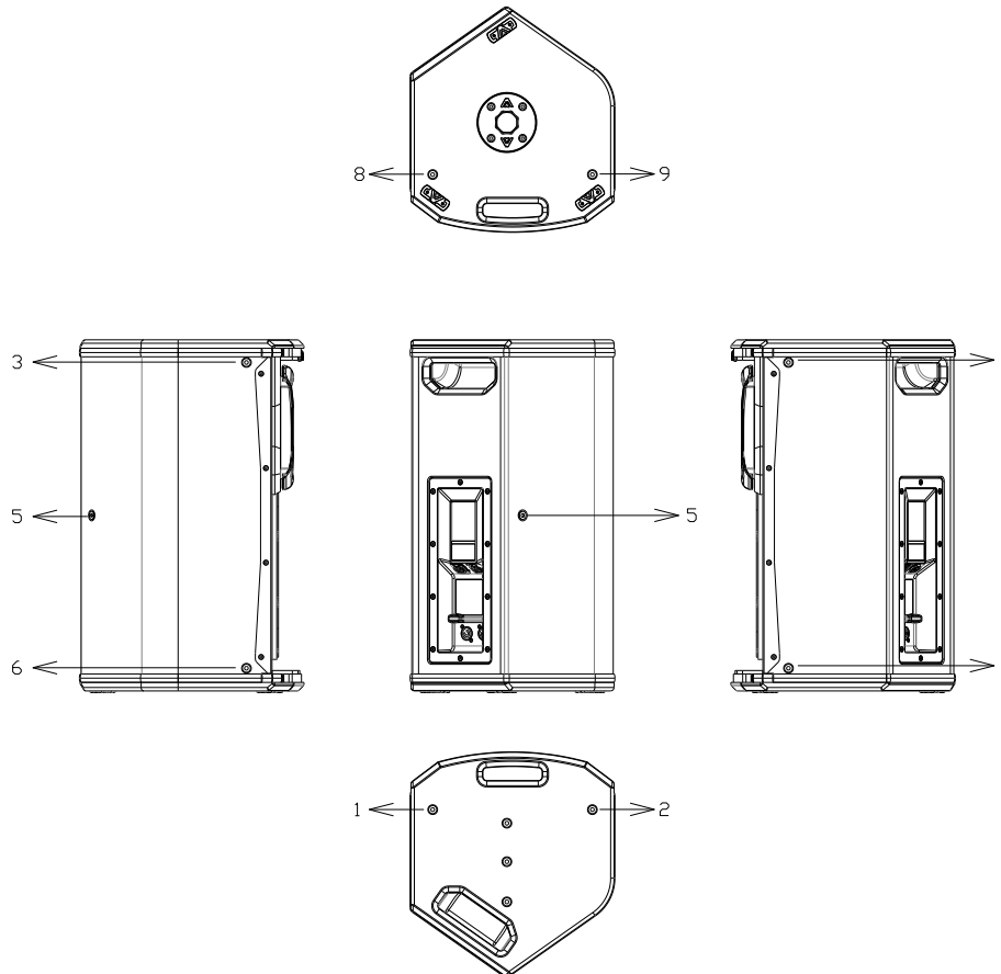
Fig. 16. Volado de una unidad S12A7 con ACR-M8
