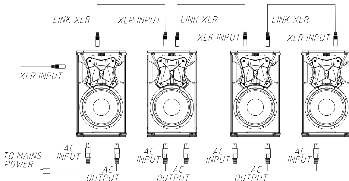
Fig. 3. Conexiones en paralelo para la S12A7
