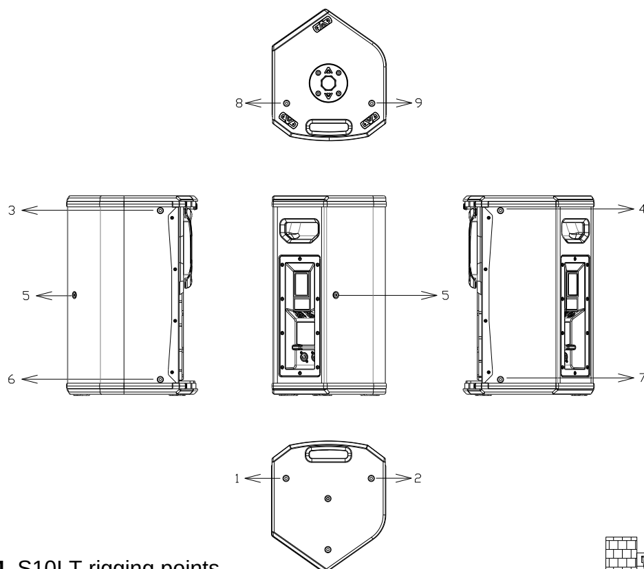
Fig. 14. S10LT rigging points
