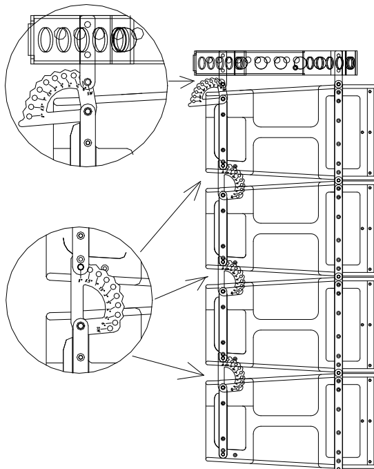
Fig.34. Volado X210. Line Array plano (Recinto 1 - Guía trasera = SW) (Recintos 2/3/4 – Guía trasera = 0^\circ )
