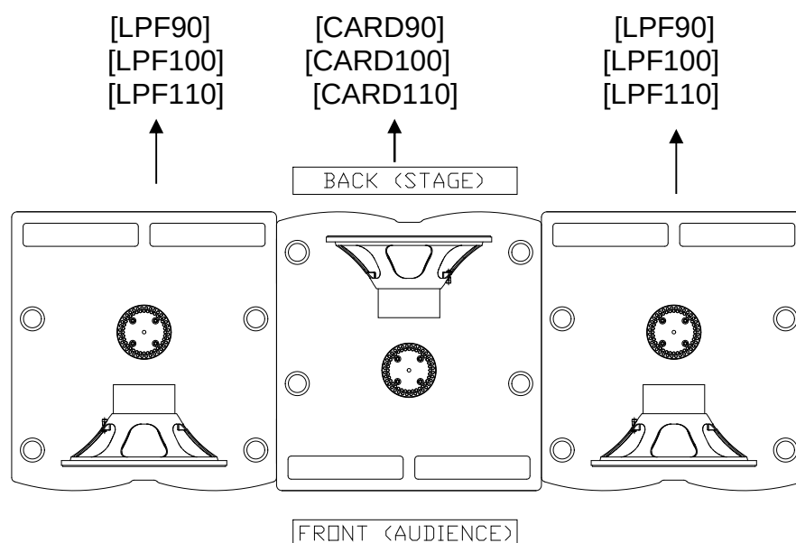
Fig.26. Presets para configuración cardioide X218W3K
