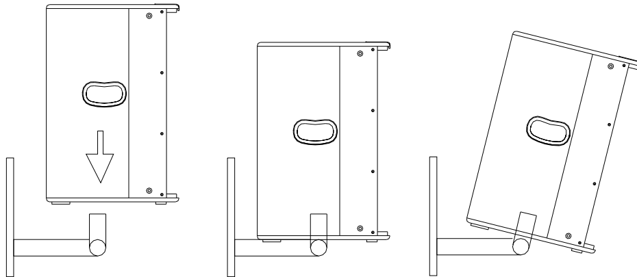
Fig.20. Soporte SP35
