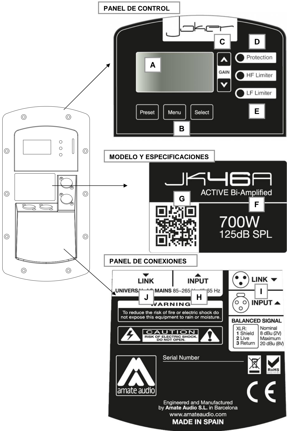
Fig.1. Panel de control y de conexiones Joker
