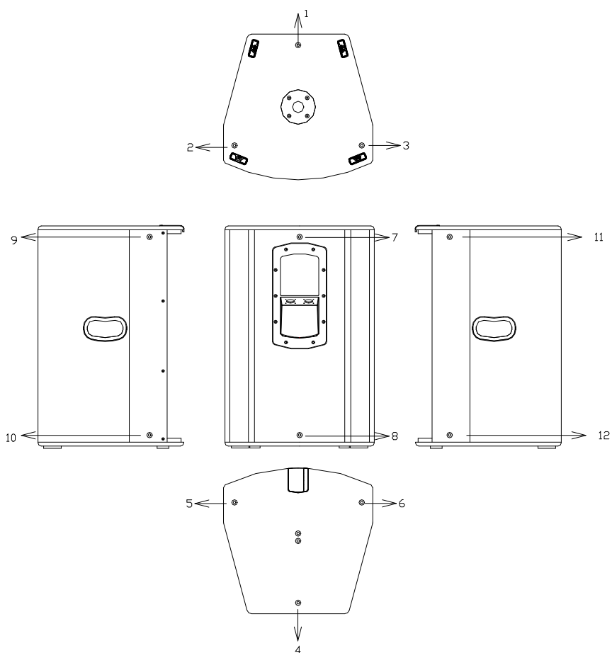
Fig.16. Puntos rigging JK15NA
