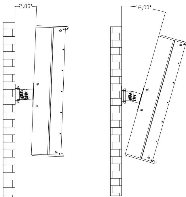
Fig.23. Soporte de pared SP46N
